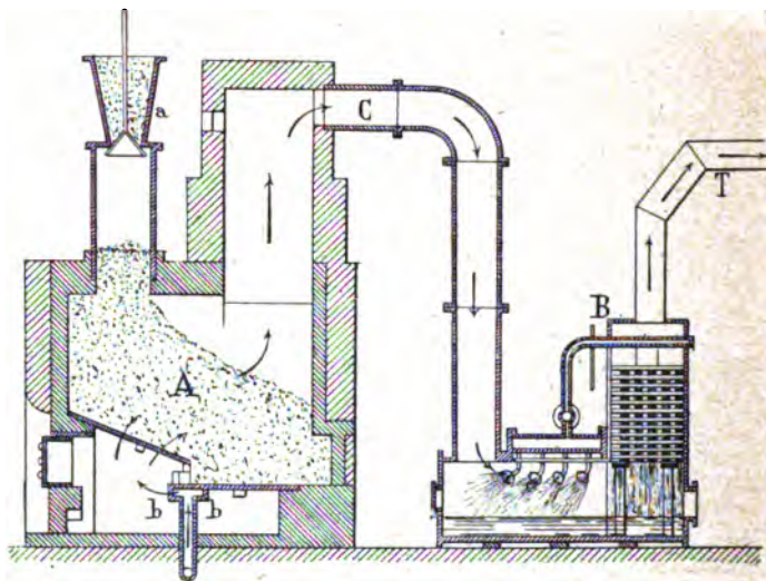
Fig. 103. — Gazogène Lundin.
